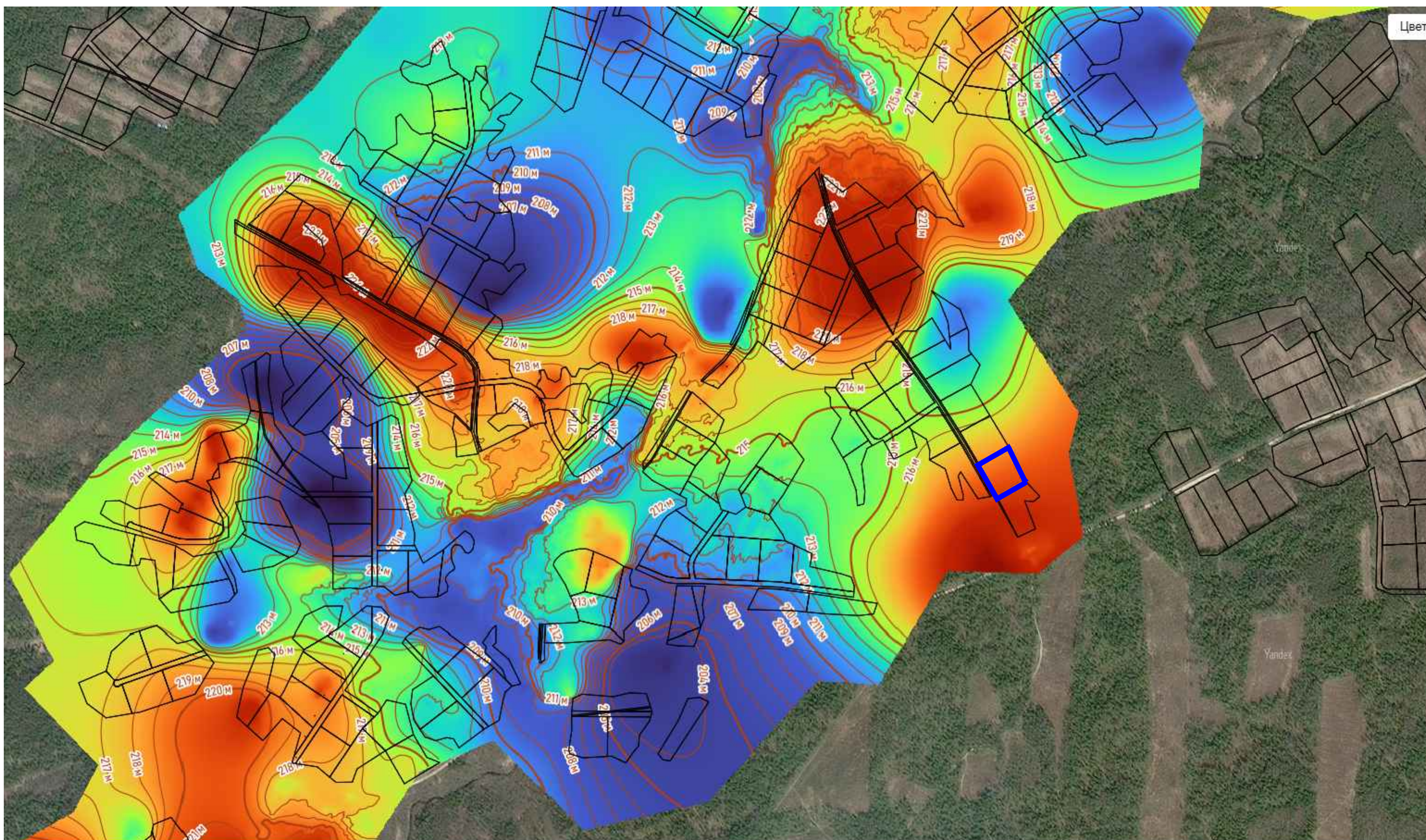
Карта высот
